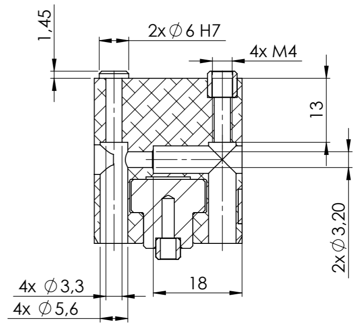
SECTION A-A SCALE 2 : 1.5
